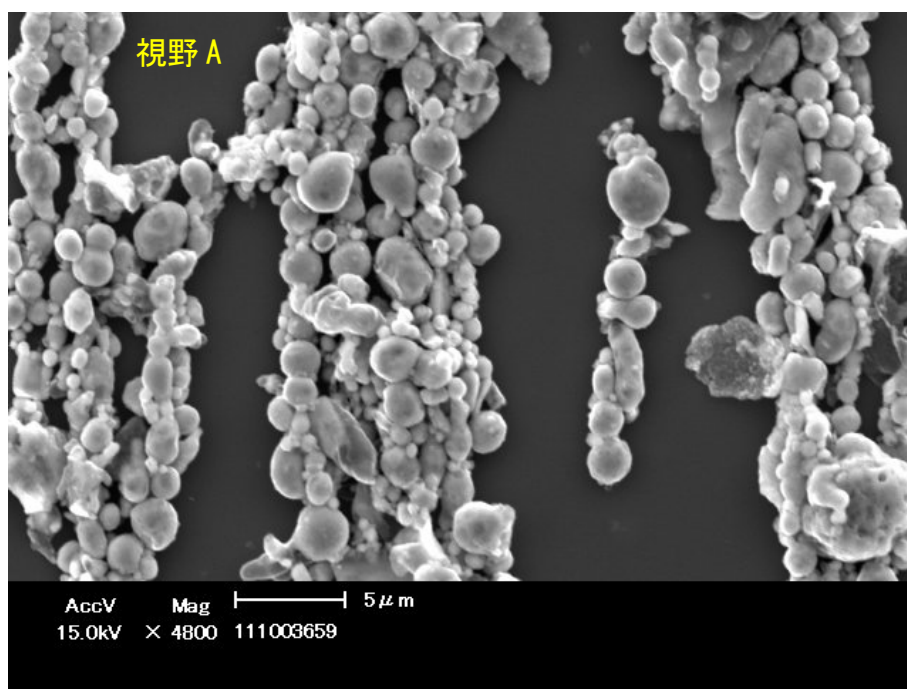
(b) 溶融摩耗粒子
