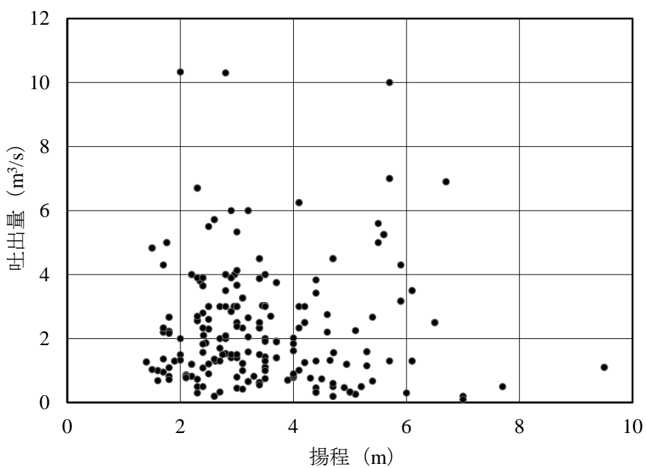
(b) 排水ポンプ設備 (1 基当たり)
