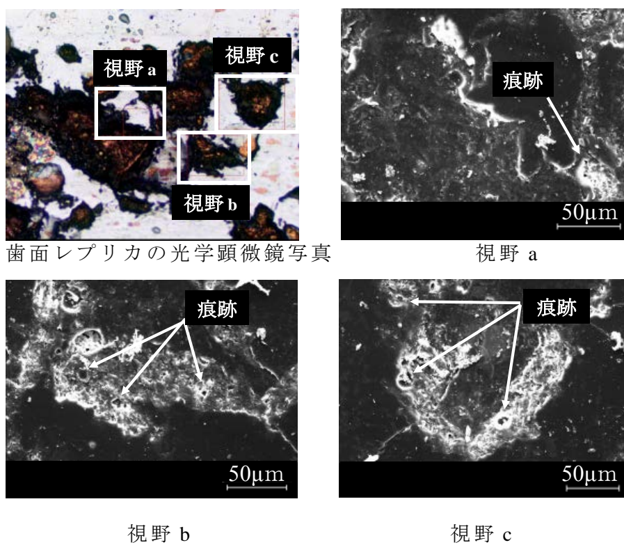
Fig. 4-14 減速機ギヤ歯面の転写レプリカ観察
