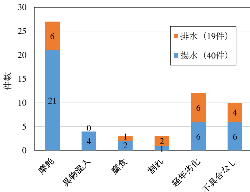
Fig. 2-8 軸受の交換理由
