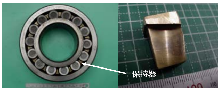
(a) ベアリングの外観
