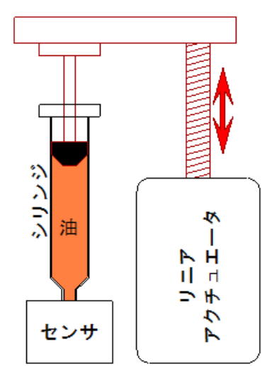
Fig. 6-4 汚染度簡易測定装置のイメージ図
