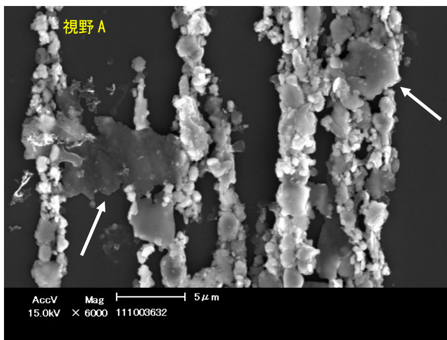
(b) 凝着摩耗粒子
