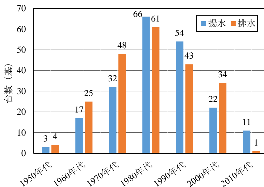
Fig. 2-5 ポンプ設備の設置年代別台数
