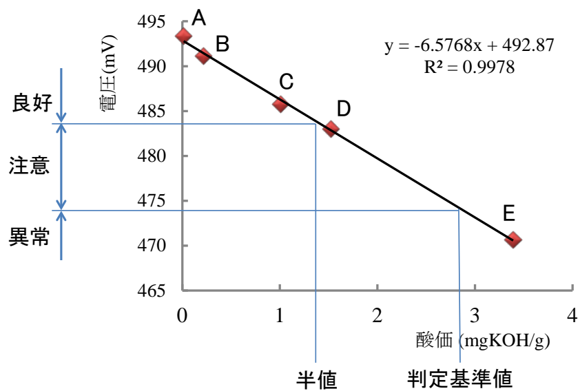
Fig. 6-2 三段階評価のイメージ図
