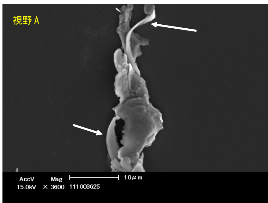
(b) アブレジブ（切削型）摩耗粒子
