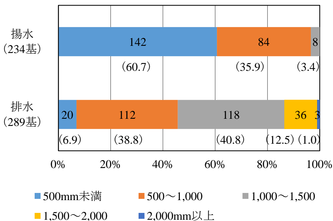
Fig. 2-3 ポンプの口径別割合
