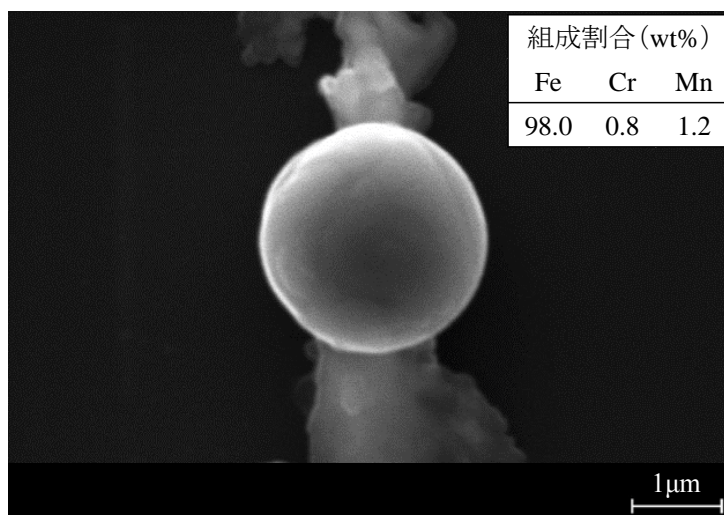
Fig. 4-12 溶融摩耗試験で確認した金属摩耗粒子
