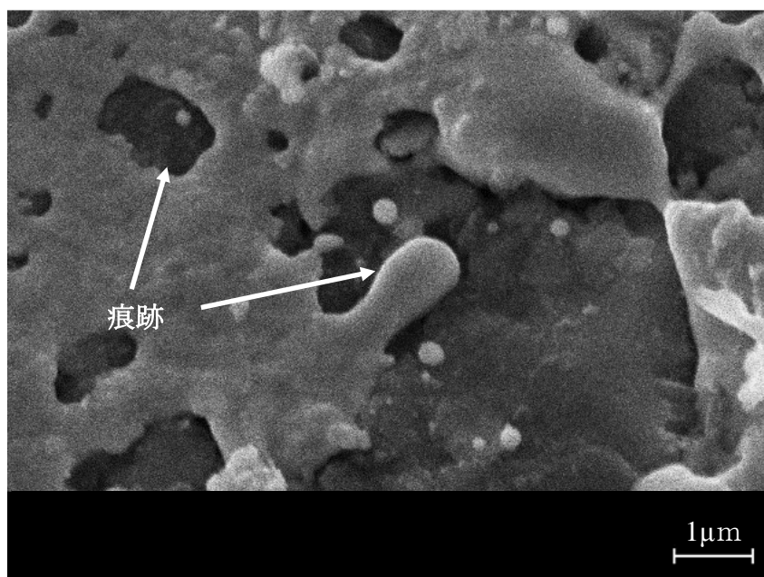
(c) 保持器軌道面の電子顕微鏡写真
