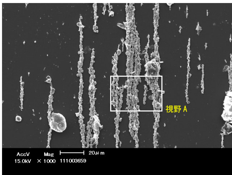
(a) 分析フェログラフィー
