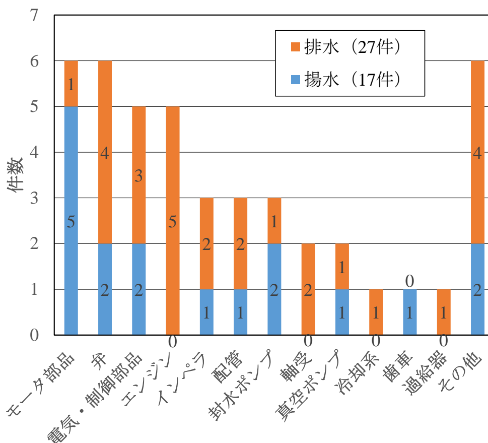
Fig. 2-10 機器の重大なトラブルの分類
