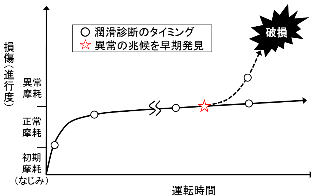
Fig. 5-10 機器の損傷進行度のイメージ図
