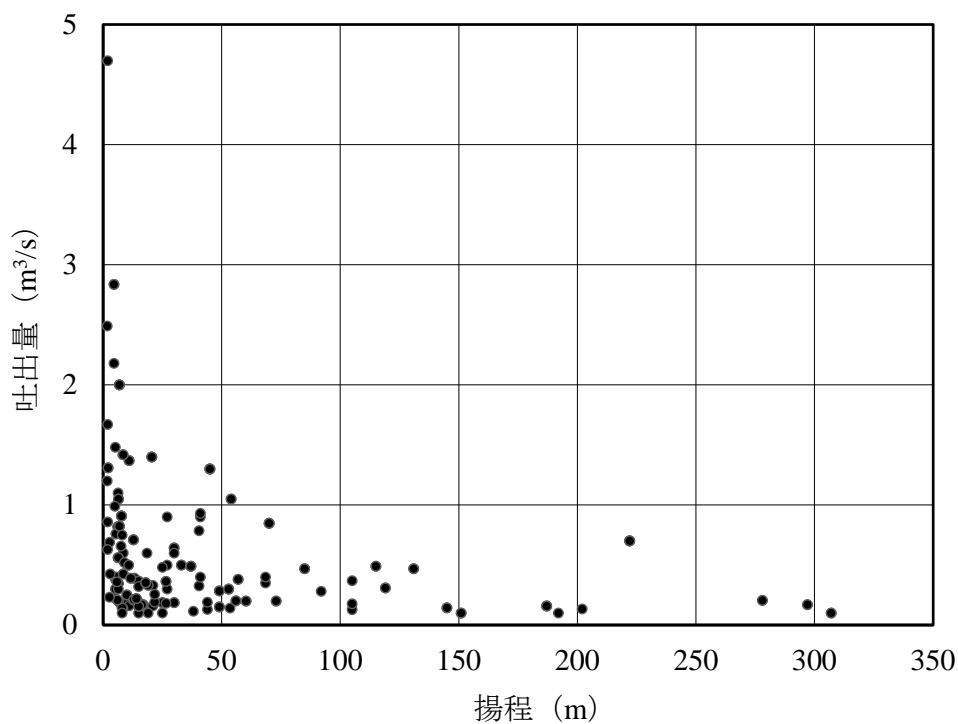
(a) 揚水ポンプ設備 (1 基当たり)
