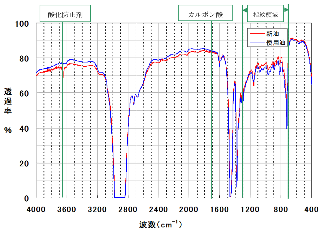
Fig. 5-3 潤滑油の IR チャート
