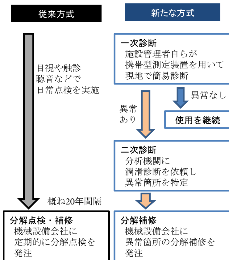
Fig. 6-8 新たな機能診断システムのフロー図
