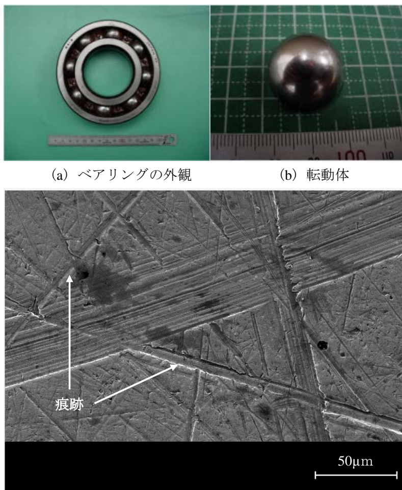
(c) 転動体表面の電子顕微鏡写真
