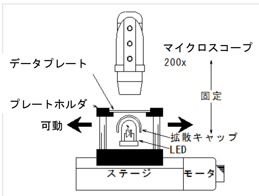
Fig. 6-6 摩耗簡易測定装置のイメージ図
