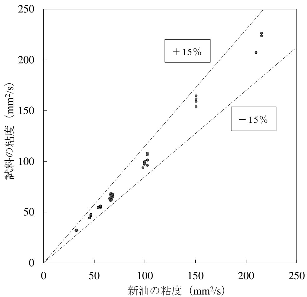
Fig. 3-2 潤滑油の粘度の変化率 (77 試料)
