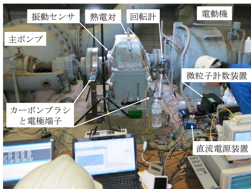
(a) 減速機に設置した測定装置
