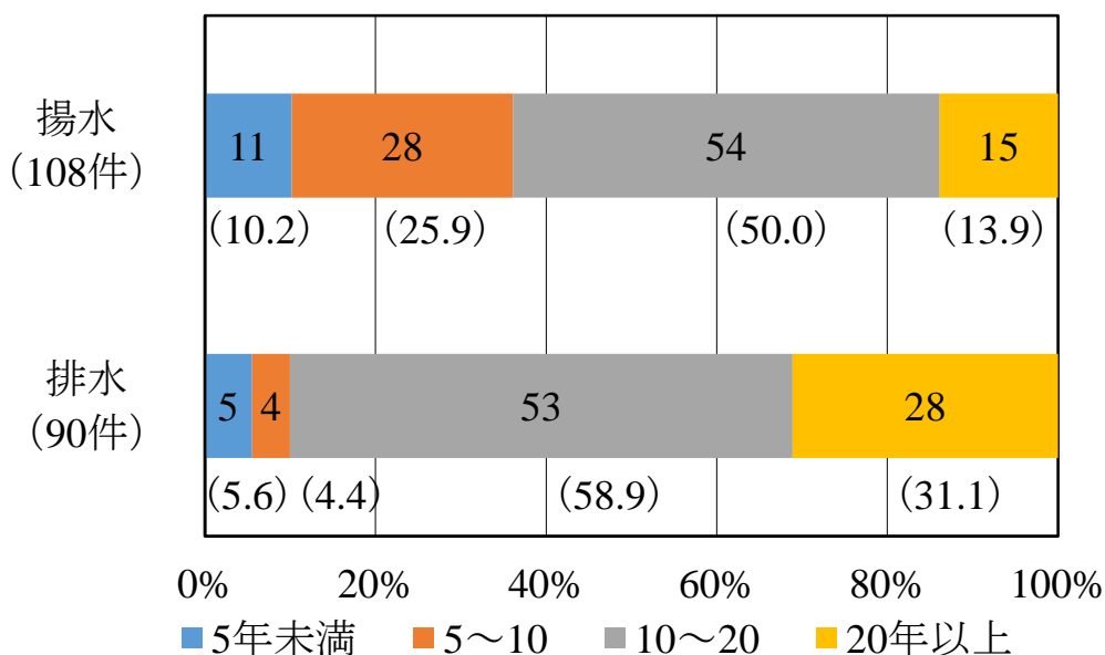
Fig. 2-7 分解点検の周期の分布
