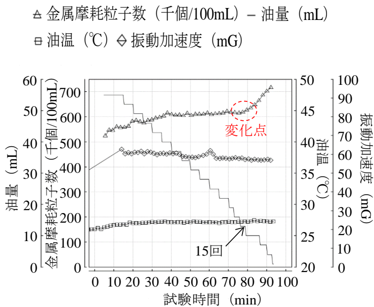
Fig. 4-8 凝着摩耗試験の測定データ Measurement data of adhesive wear test
