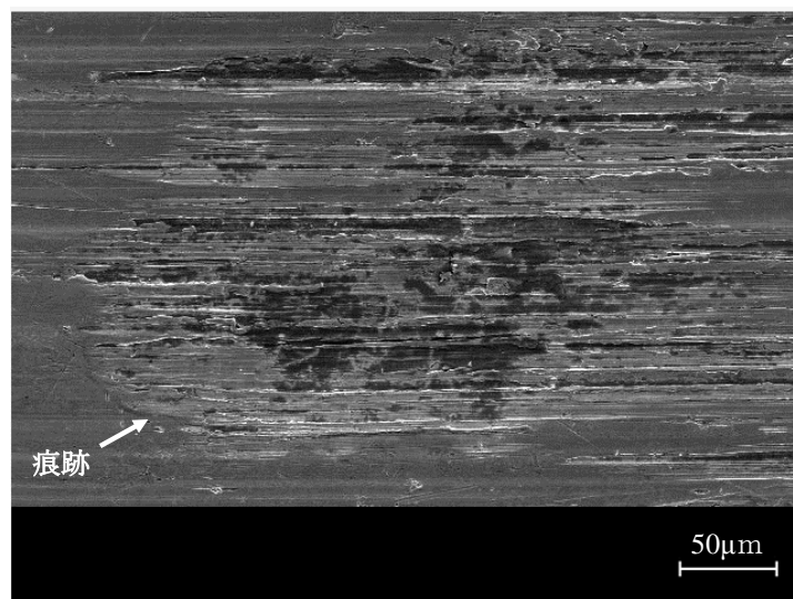
(c) 軸表面の電子顕微鏡写真
