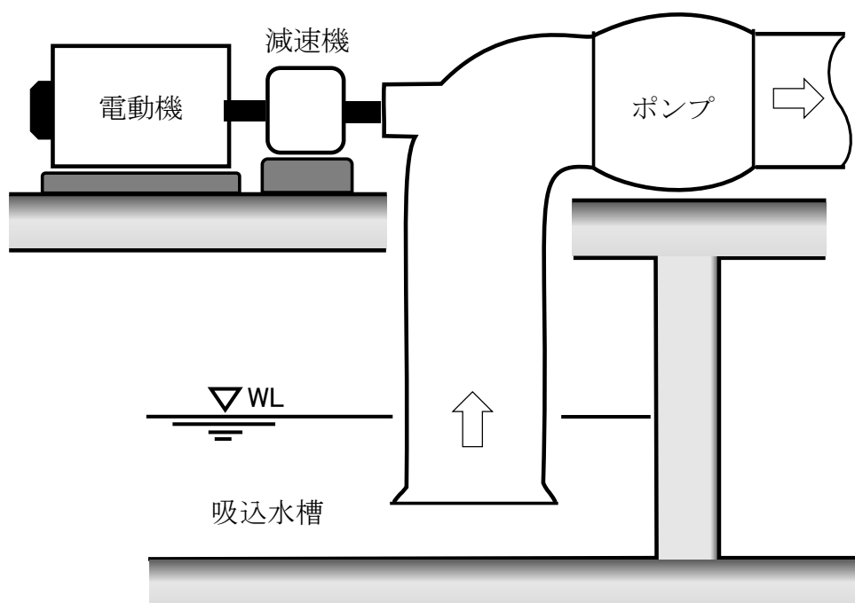
(b) 構造図
