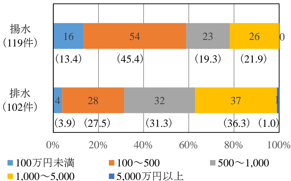
Fig. 2-6 分解点検の概算費用の分布 (1件当たり)
