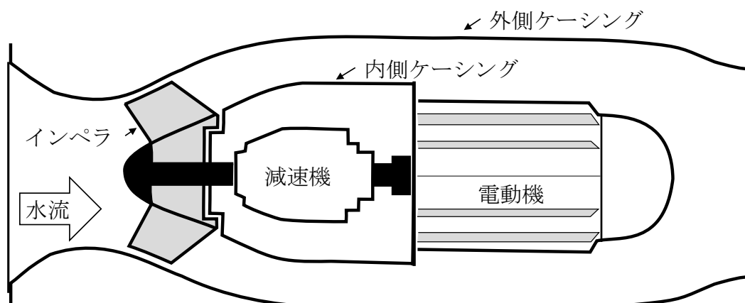
(b) 構造図 (断面図)
