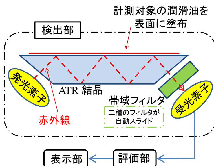
Fig. 6-1 劣化簡易測定装置のイメージ図
