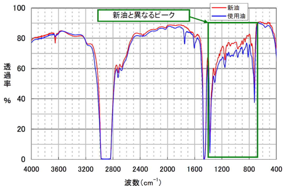
Fig. 3-1 潤滑診断の IR チャート（一例）
