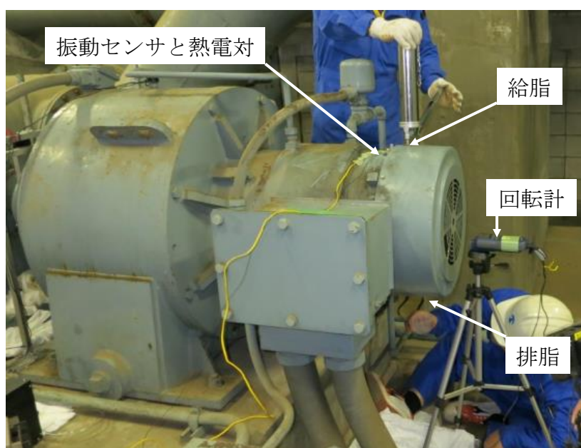
Fig. 4-2 電動機軸受を対象としたアブレイブ摩耗試験 Abrasive wear test for the bearing of motor
