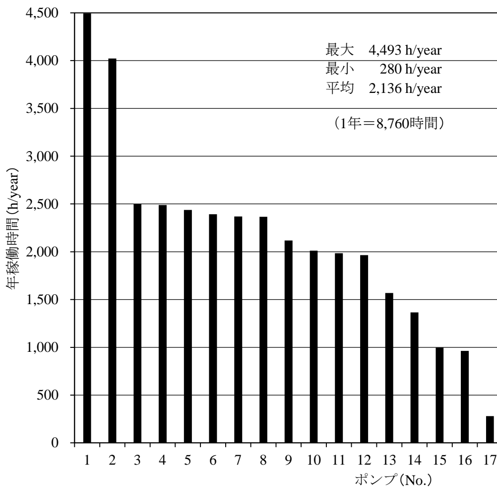
Fig. 1-2 農業用揚水ポンプの稼働実績
