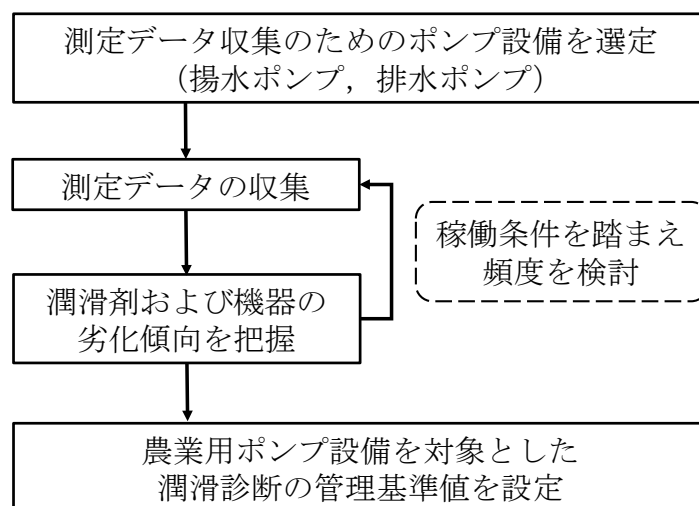
Fig. 5-11 管理基準値の設定のためのフロー図
