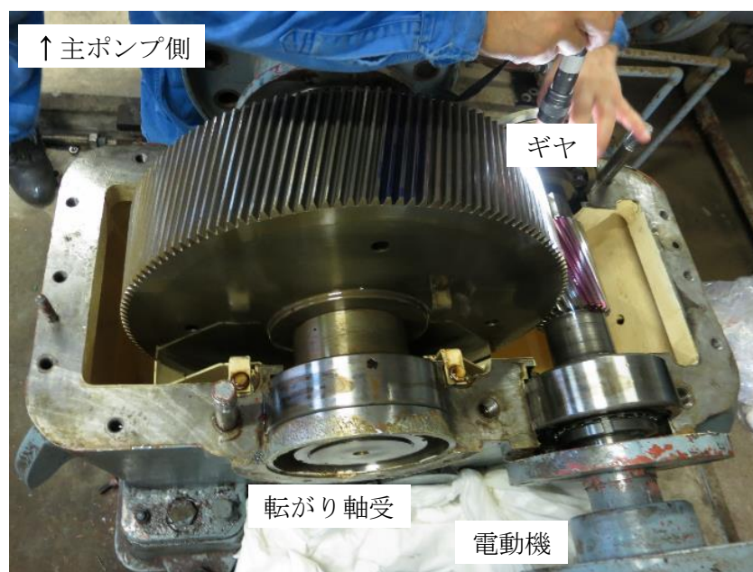
(b) 減速機の内部
