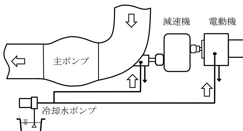
(b) ポンプ設備の構成
